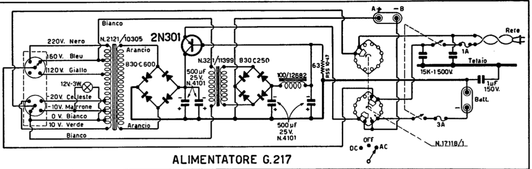
Schema elettrico alimentatore G 217
